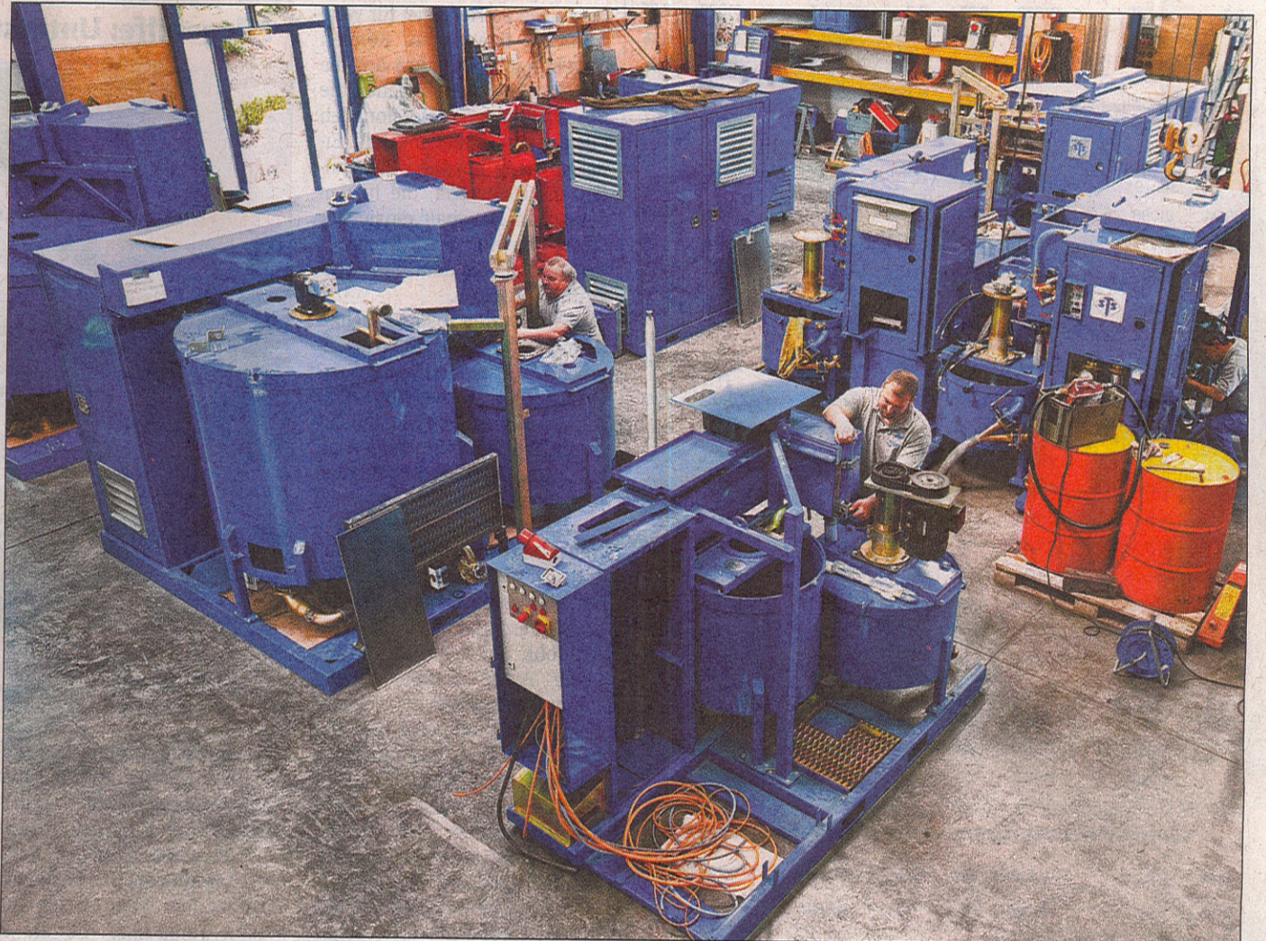
Auf Entwicklung und Montage von Misch-Pump-Stationen für die Tiefbau-Branche ist die Firma Scheltzke spezialisiert.
